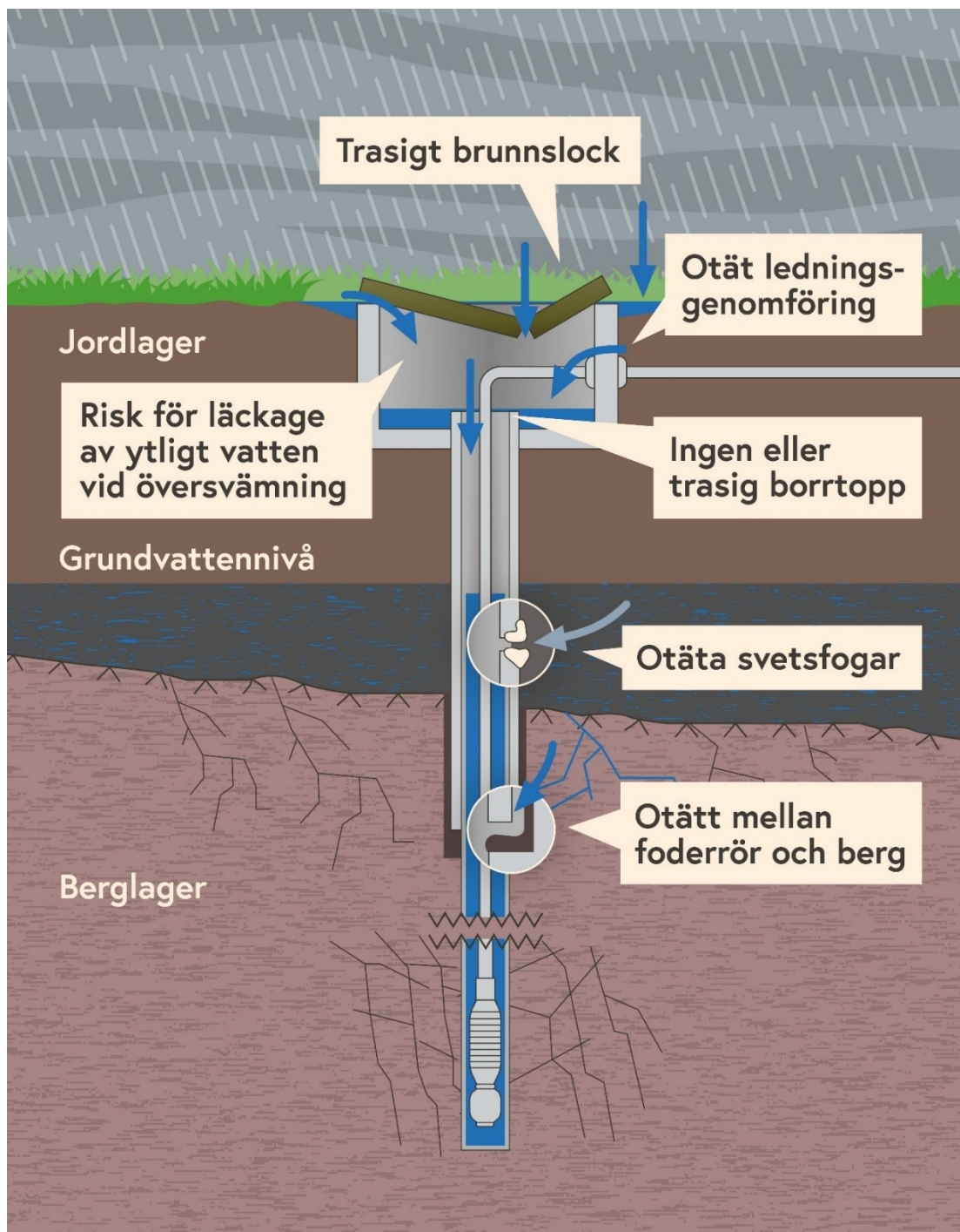
Figur 16. Kritiska punkter i bergborrade brunnar. De blå pilarna illustrerar ställen där yttligt vatten kan tränga in och förorena brunnen.
