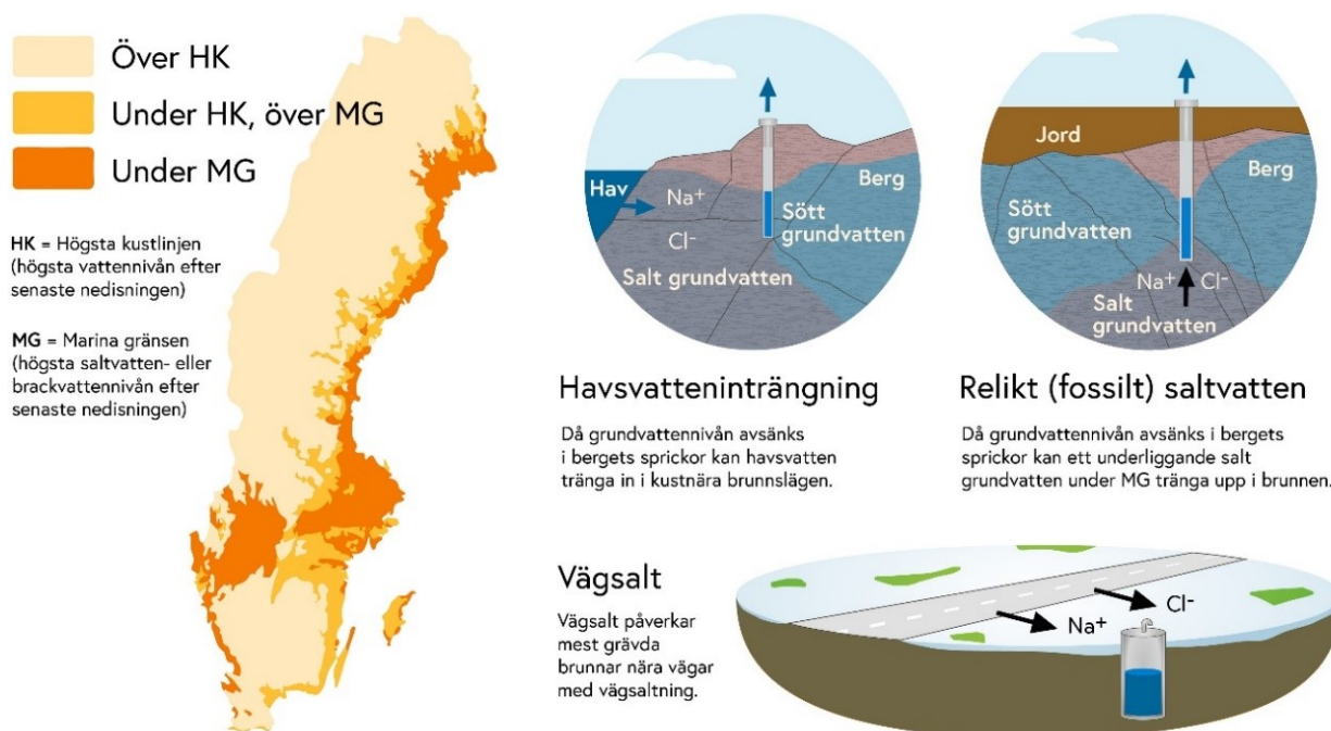
Figur 12. Vanliga orsaker till salt grundvatten i brunnar. Detta kan vara till exempel havsvatteninträngning i kustnära områden, relik saltvatten under den marina gränsen (MG) samt vägsalt. Kartan visar områden i Sverige som varit täckta av havsvatten och där det kan finnas relik salt grundvatten.
