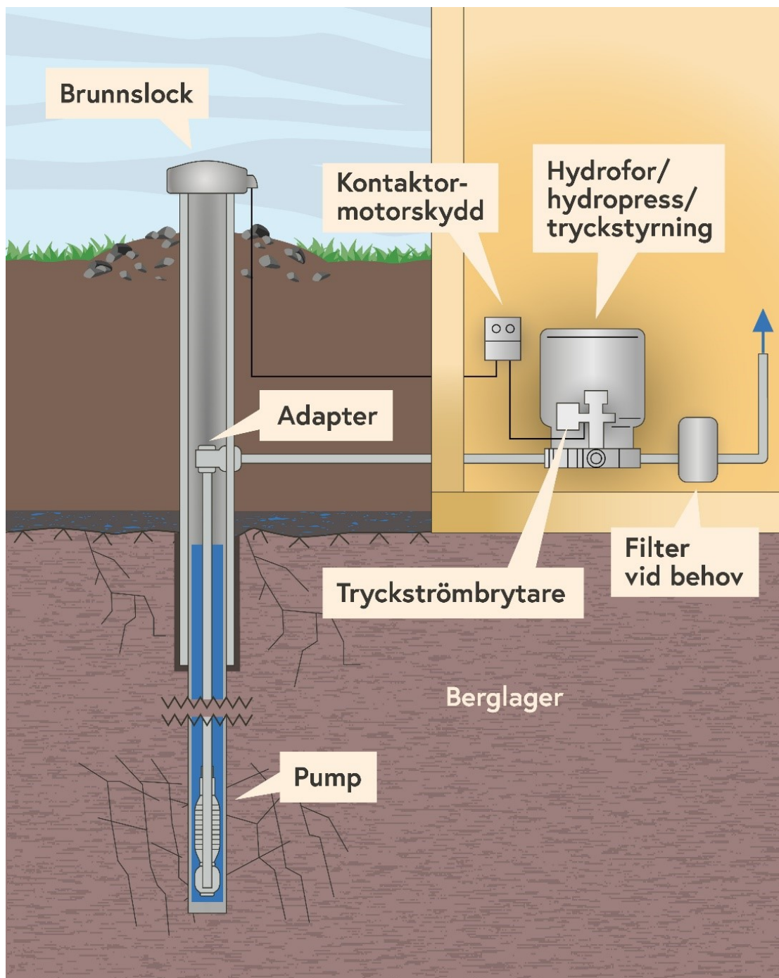
Figur 9. Exempel på hur installationer för en bergborrad brunn med sänkpump kan se ut.
